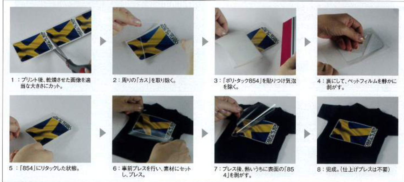
「ポリ・フレックス プリンタブル 4036 ターボ」の転写工程
