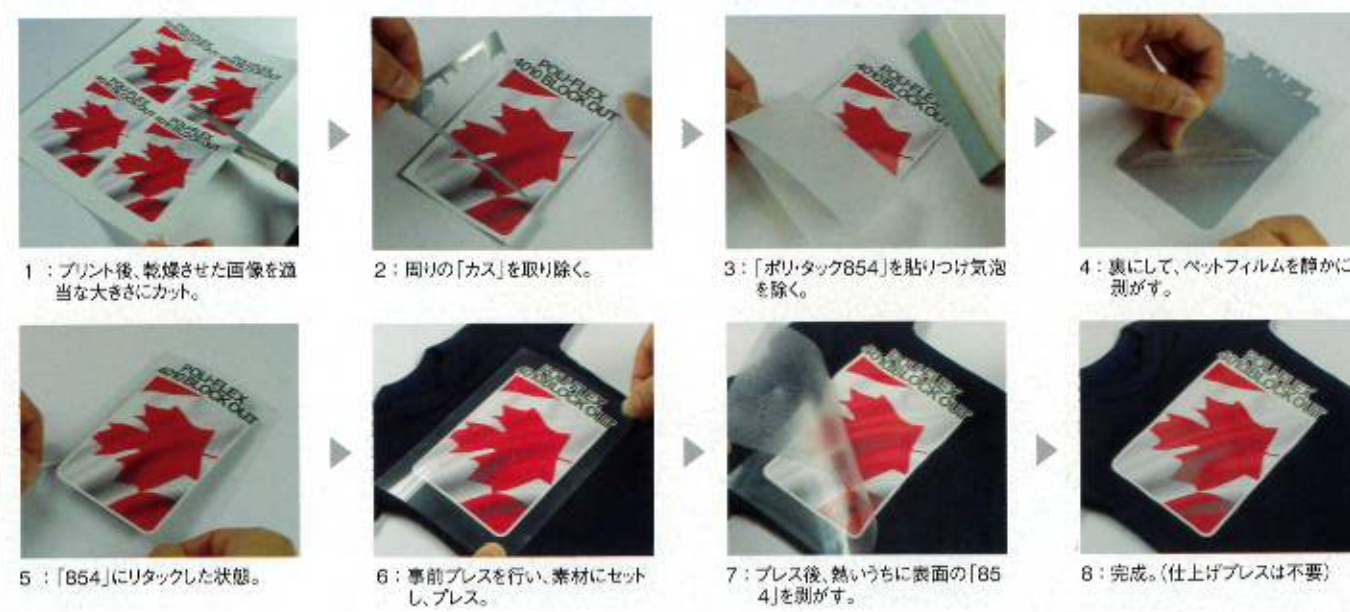
「ポリ・フレックス プリントابل 4010S ブロックアウト」の転写工程
